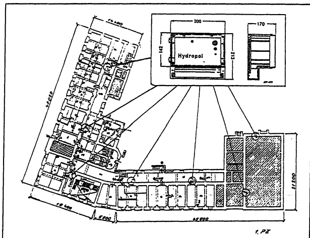
Metoda odvlhčení: Hydropol Objekt: Slovanské gymnázium Olomouc, třída Jiřího z Poděbrad 13 Datum montáže zařízení: 24. 8. 1995
