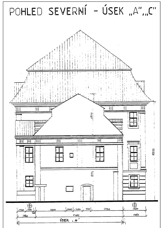
Ing. arch. Pavel Chadraba: Rekonstrukce vnějšího pláště Vincentina na Velehradě (2000) - pohled severní, úsek A a C, č. výkresu 6
